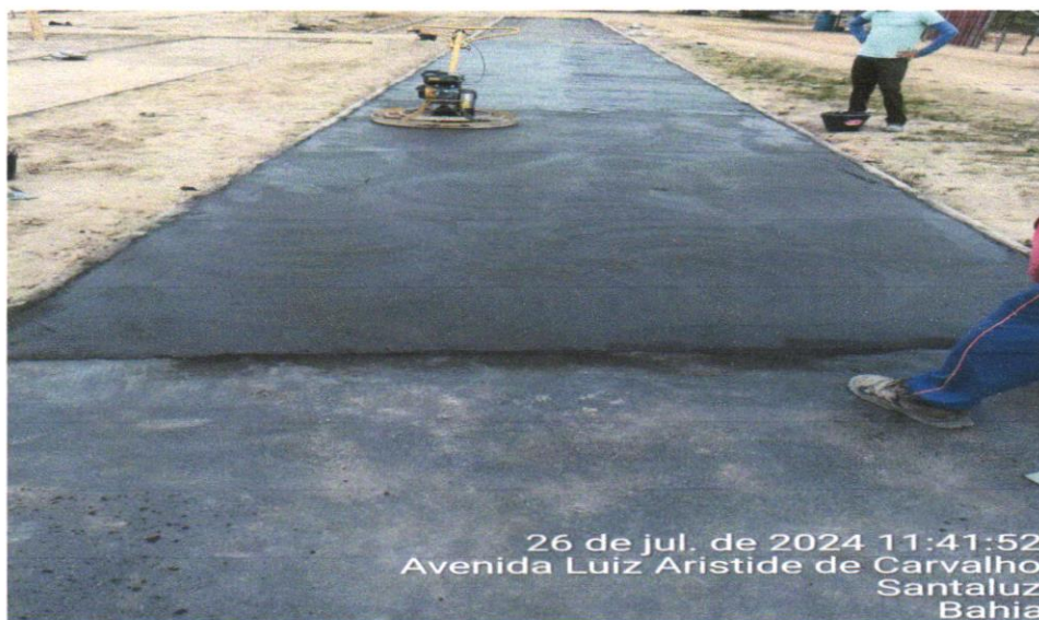
FOTO 01 – PAVIMENTAÇÃO EM CONCRETO, COM ESPESSURA DE 7 CM, COM ACABAMENTO FEITO UTILIZANDO ALISADORA DE CONCRETO (HELICOPTERO), INCLUIDO TELA DE AÇO SOLDADA NERVURADA CA60, Q196 (3,11 KG/M2), DIAMETRO DO FIO 5.0 MM, LARGURA = 2,45 M, ESPAÇAMENTO DA MALHA = 10 X 10 CM, JUNTA DE DILATAÇÃO EM PVC A CADA 2,00 M, CONCRETO FCK = 20 MPA
